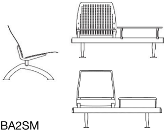
BA2SM w49" d28.5" h33" sh17"
